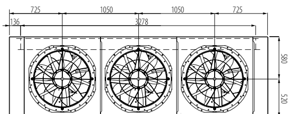
Mod. MC 352-P÷372-P MC/SL 352-P÷372-P MC/SSL 232-P÷272-P÷302-P
