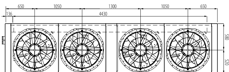
Mod. MC 352-P÷372-P MC/SL 352-P÷372-P MC/SSL 232-P÷272-P÷302-P
